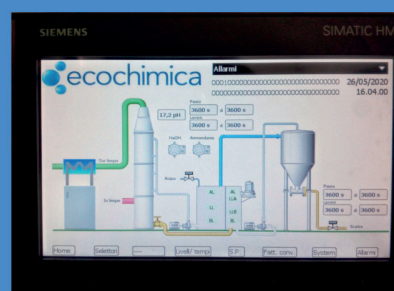
Fig.4 Sistema di automazione (PLC) Automation system (PLC)
