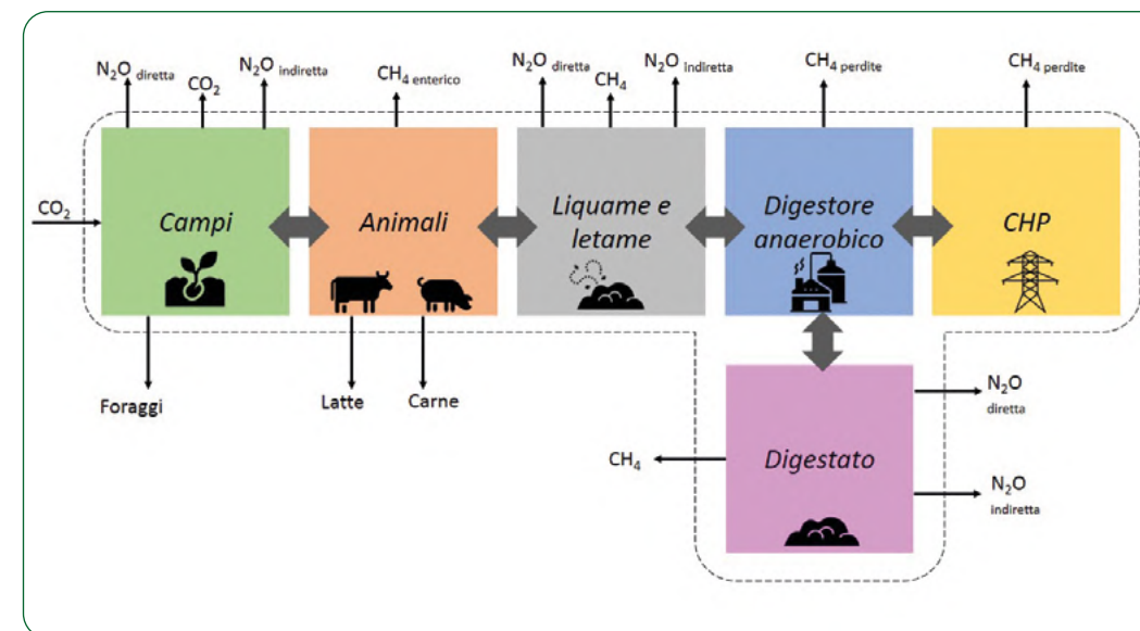
Figura 1: I confini del sistema per lo studio LCA delle aziende agro-zootecniche con impianto di biogas Figure 1: Limits of the system for LCA study of farms with biogas plant.
