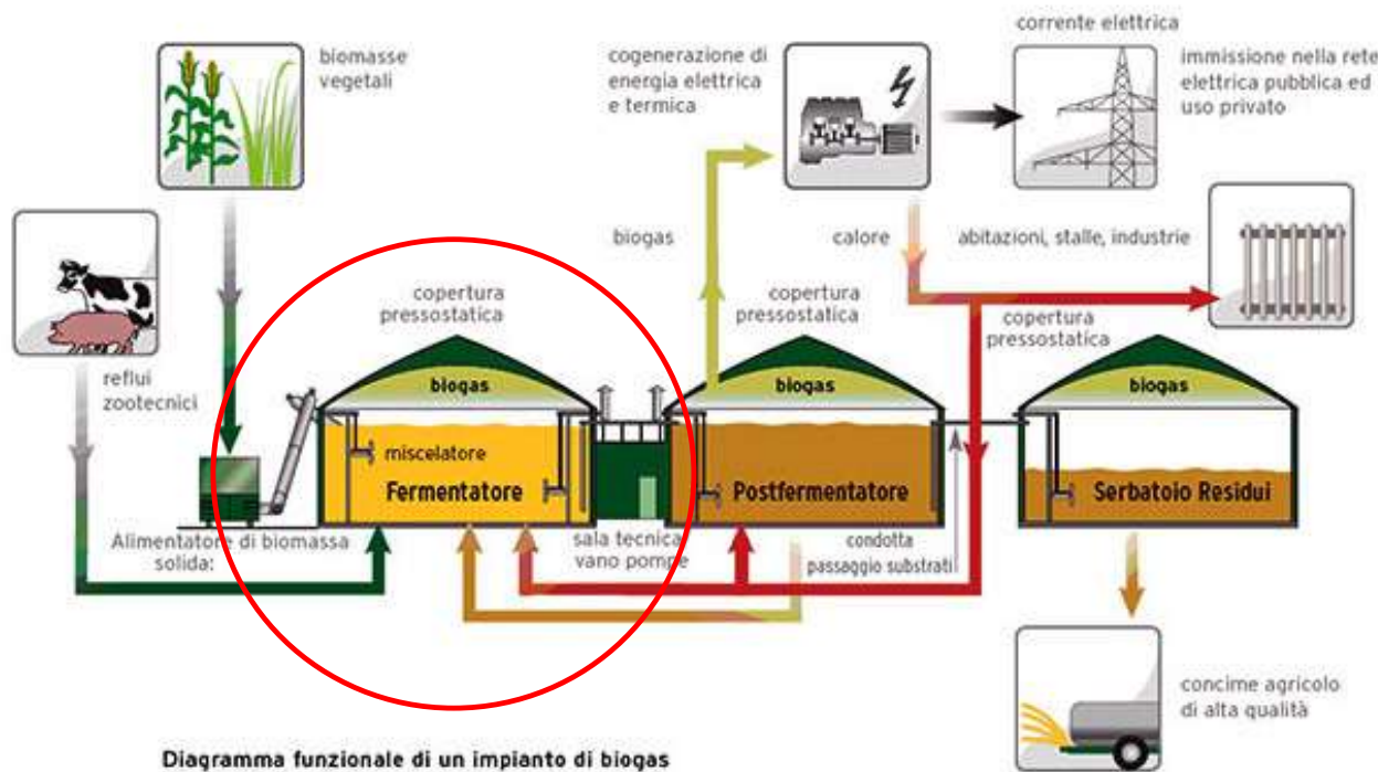
Diagramma funzionale di un impianto di biogas
